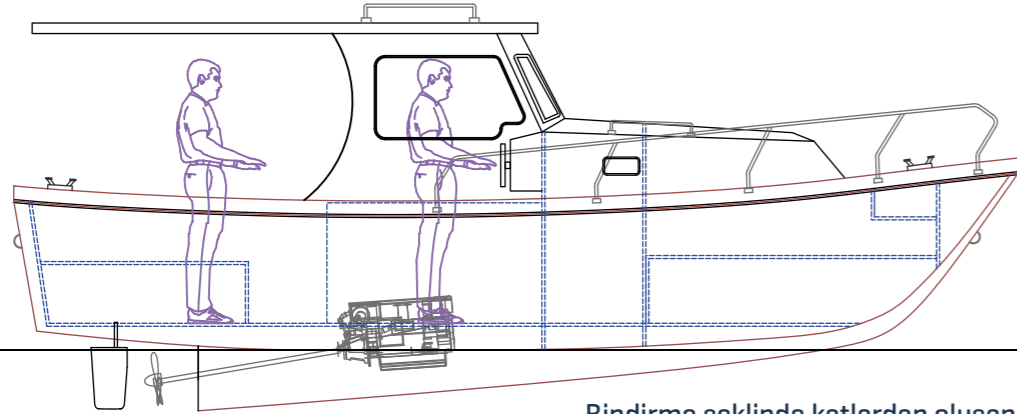
Bindirme şeklinde katlardan oluşan gövde yapısı Hull Form
